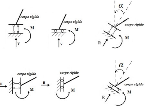
Doppio Pendolo o bipendolo
