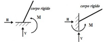
Incastro
